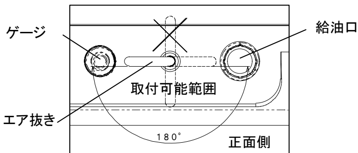
ホームタンクを上から見た図
