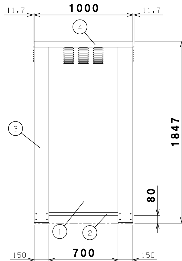
背面図
