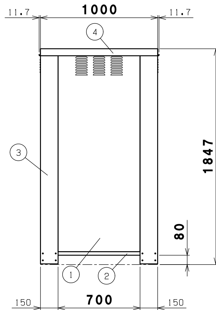
背面図
