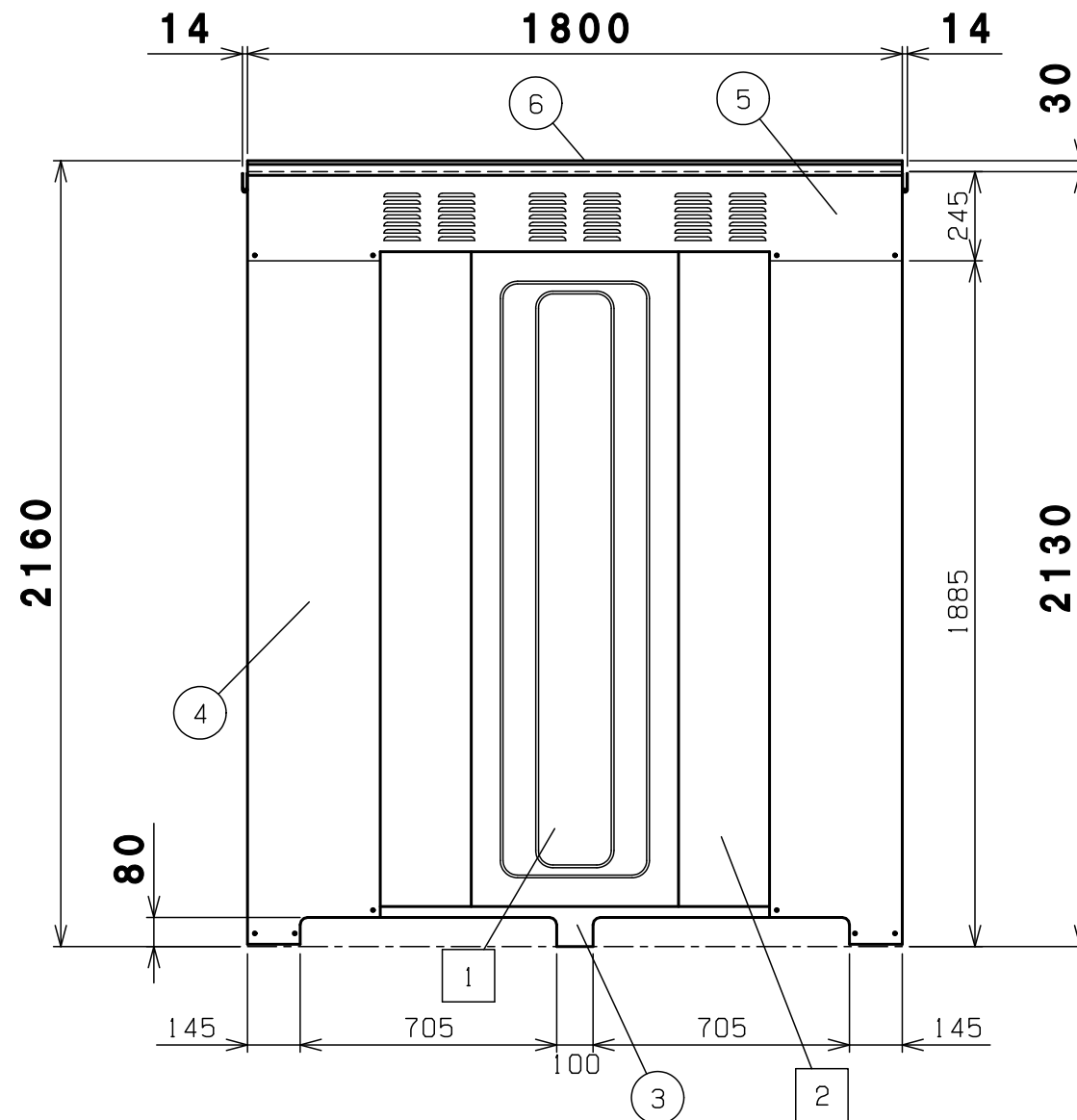
背面図
