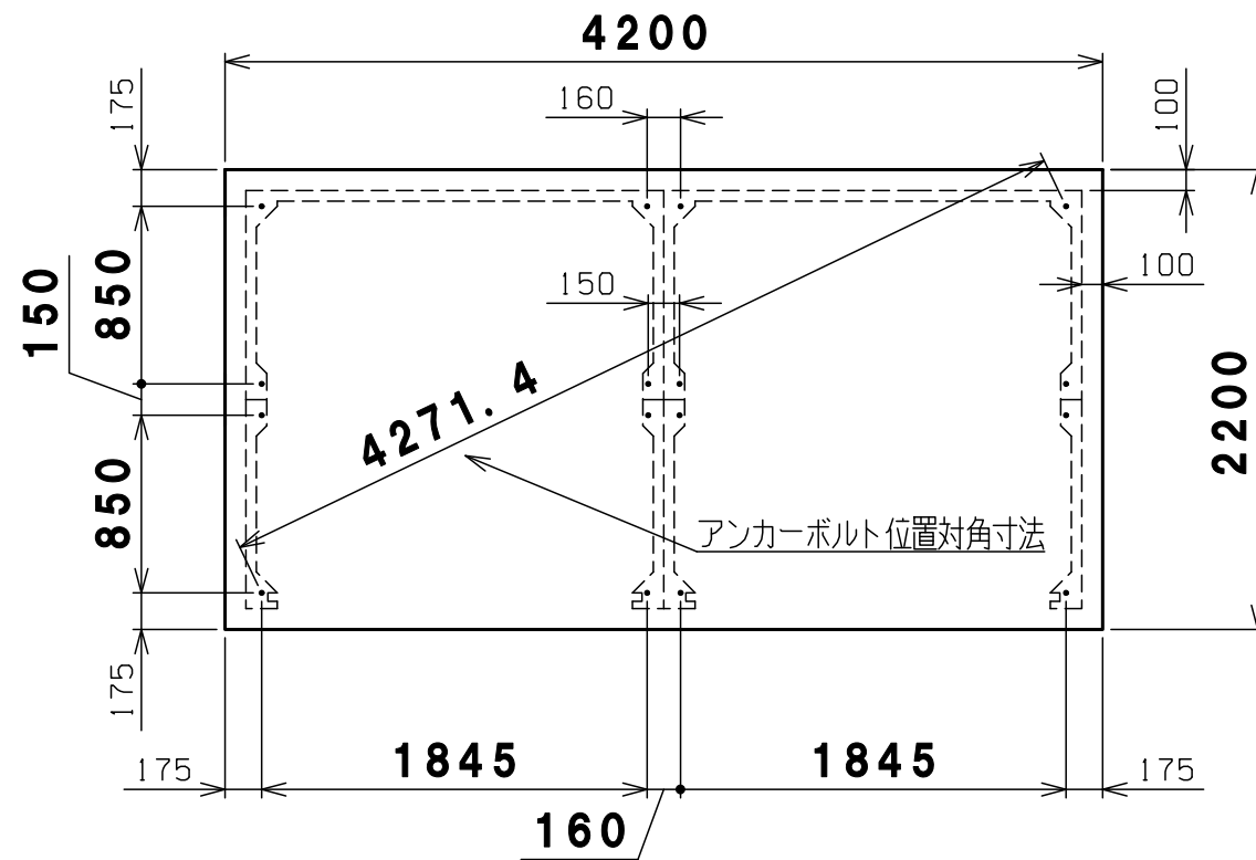
基礎平面図
