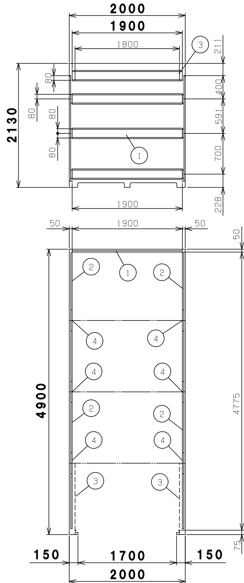
内面図
