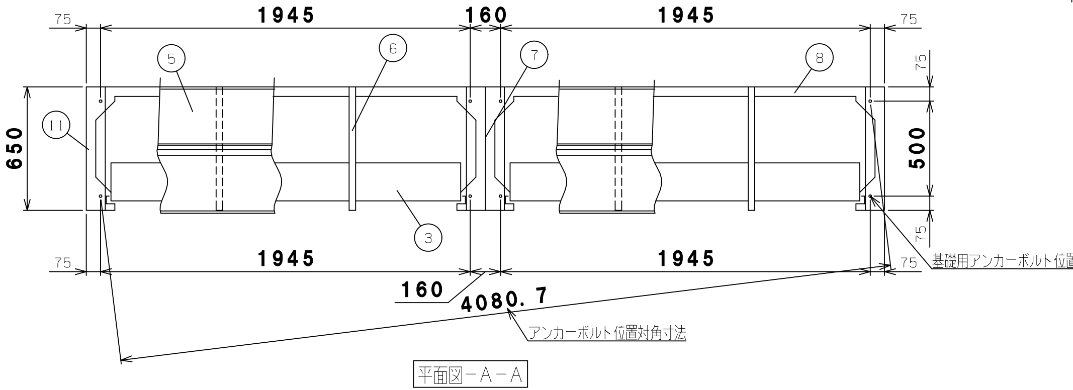
防火設備 (乙種防火シャッター仕様)
