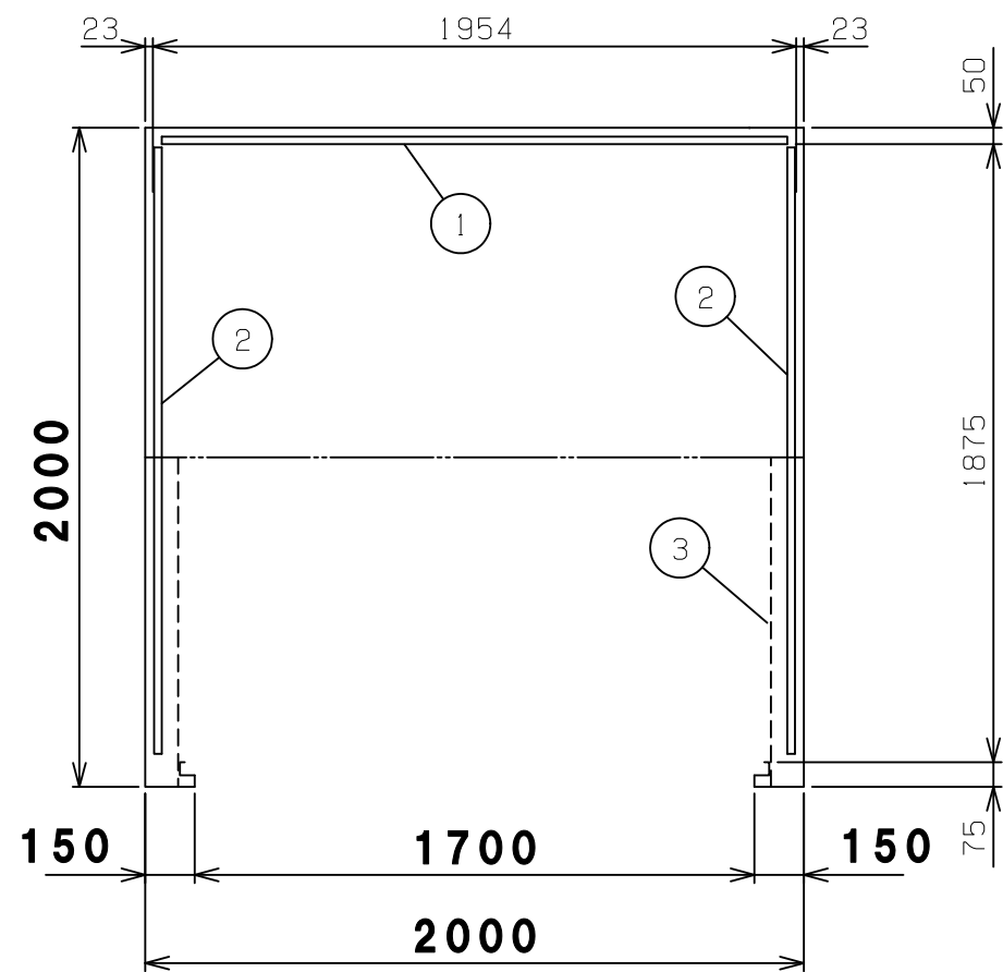
内面図
