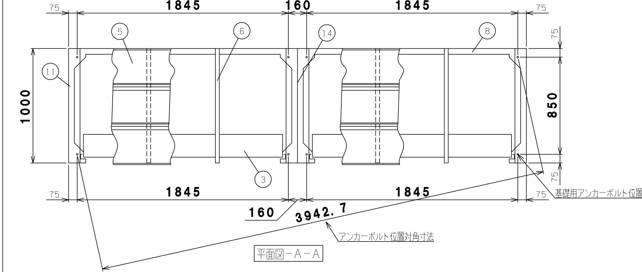
防火設備 (乙種防火シャッター仕様)
