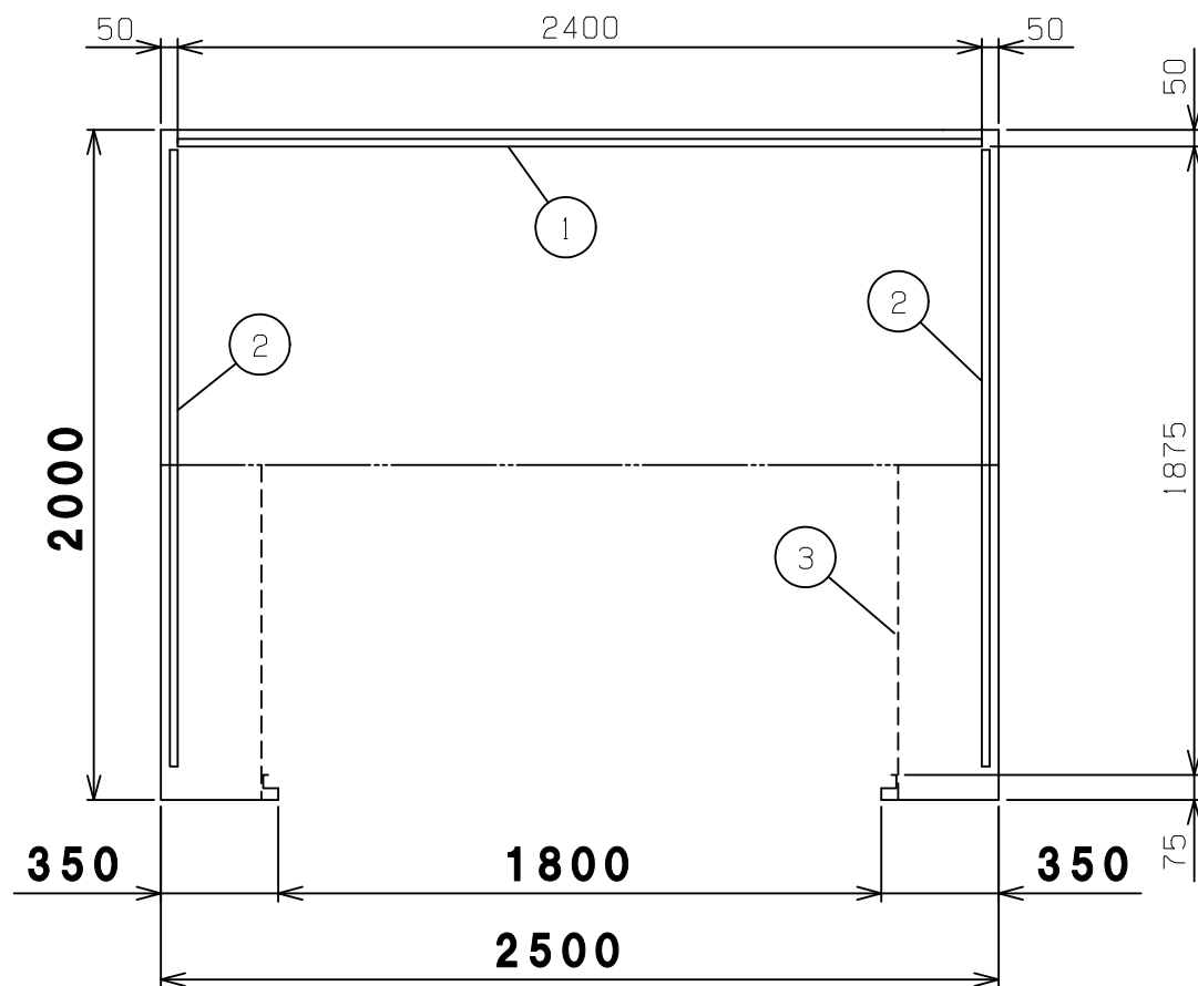
内面図
