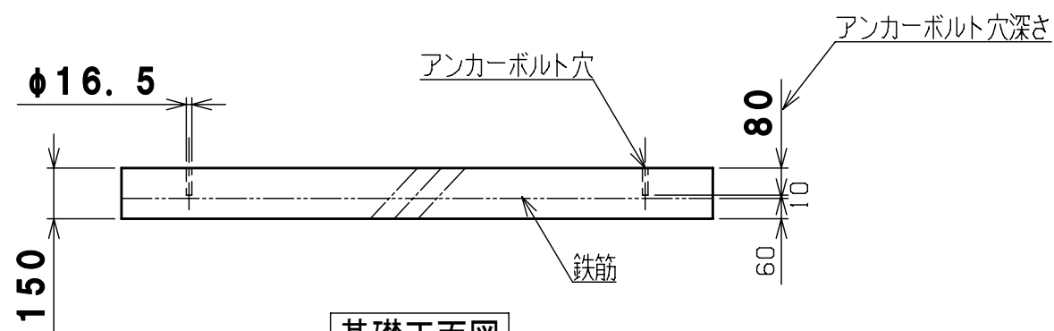
基礎正面図
