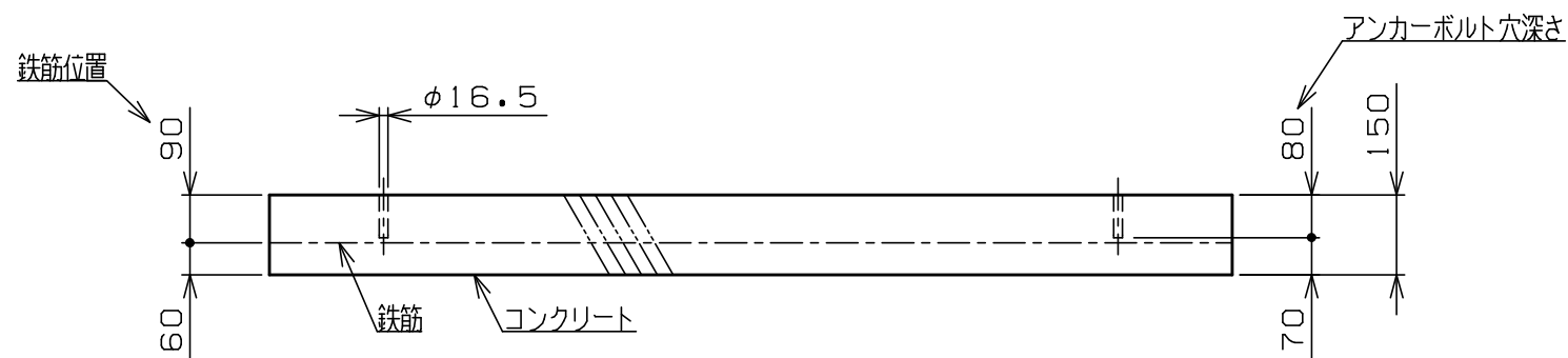
基礎土台図
