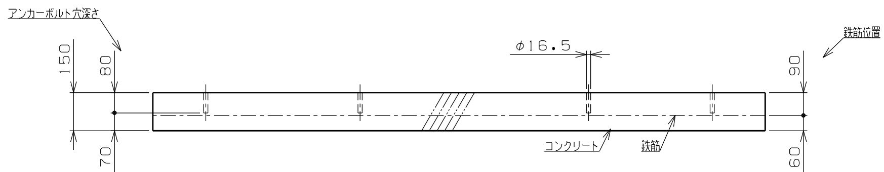
基礎土台図
