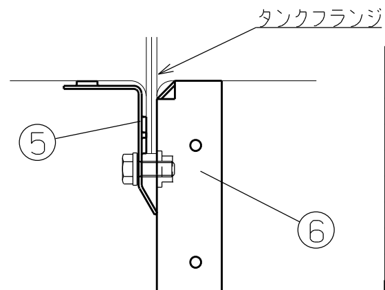
ホームタンクへの取り付け部詳細
