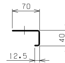
脚 断面形状
