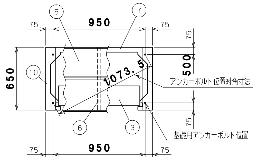
平面図-A-A
