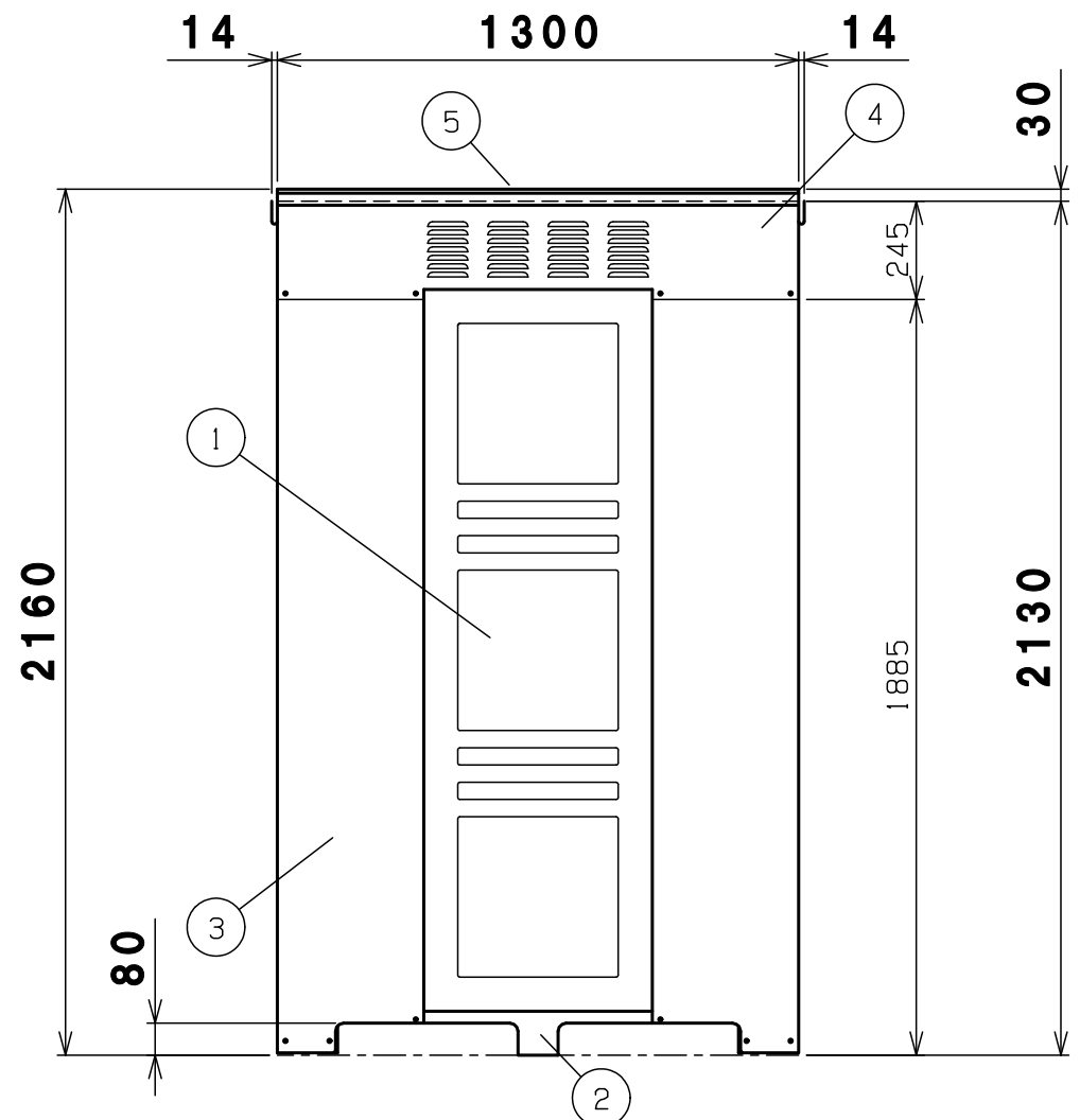
背面図
