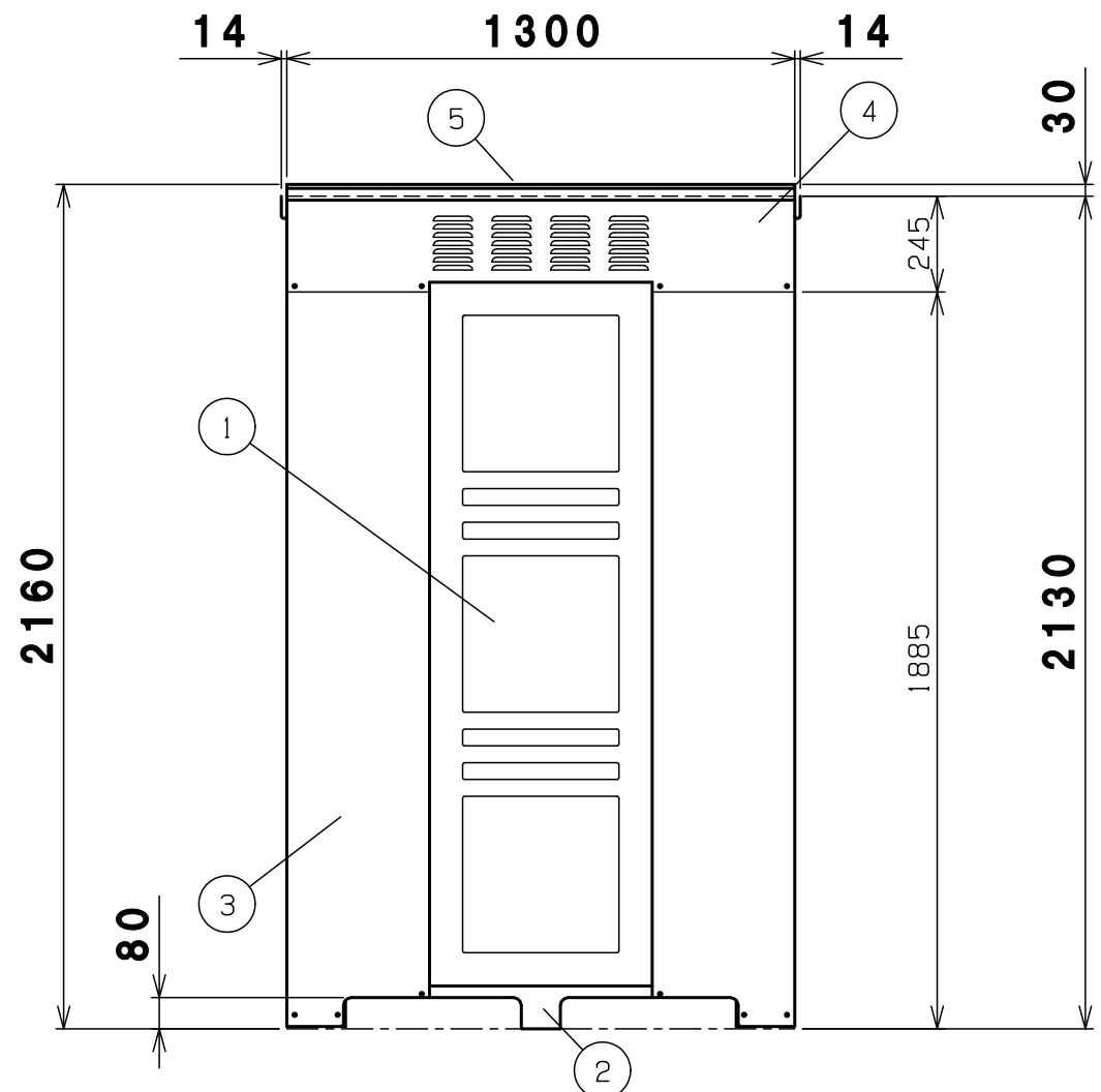
背面図
