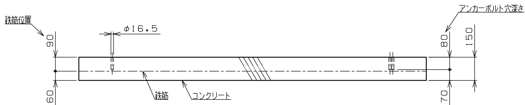
基礎土台図
