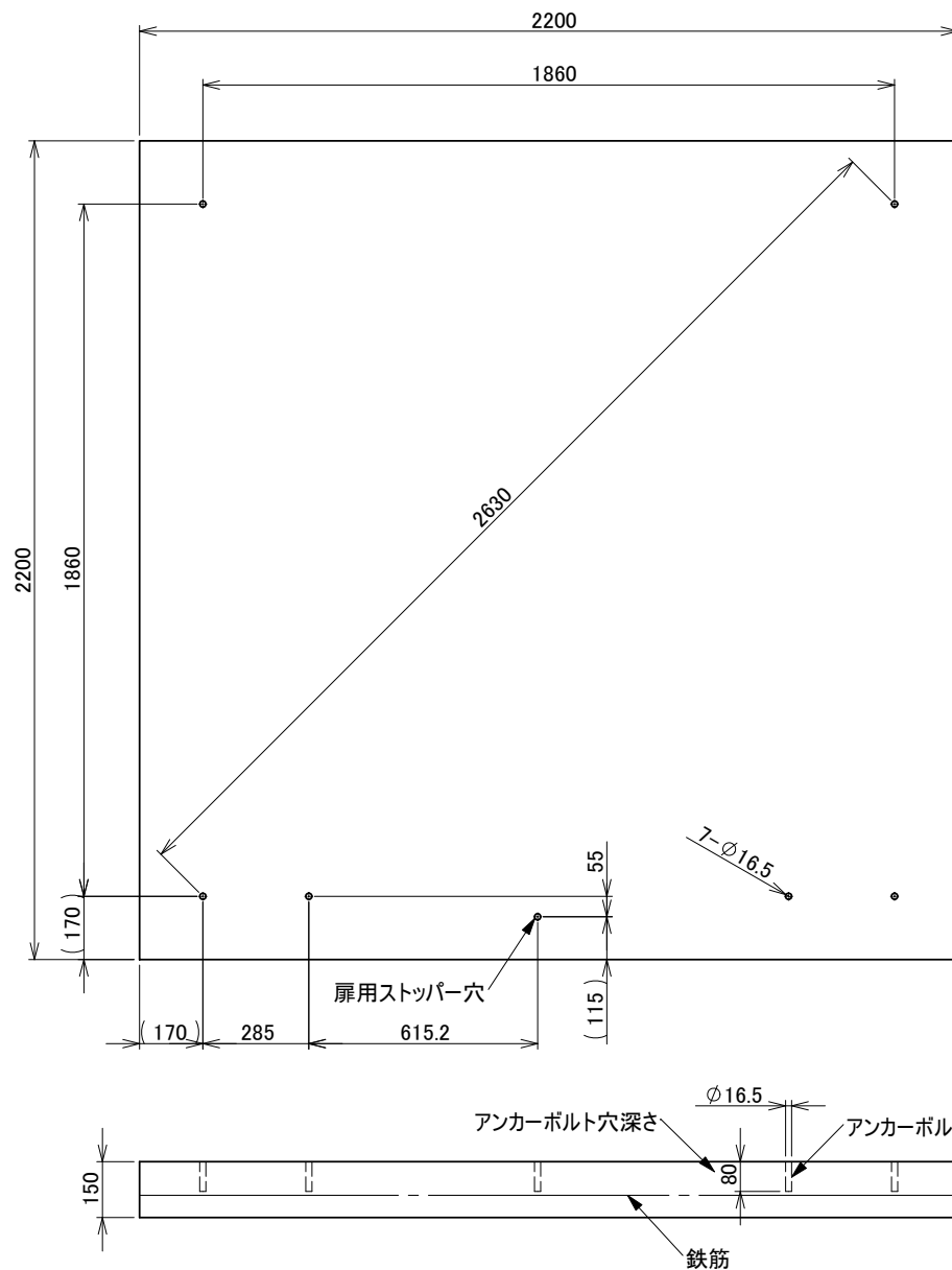
承認図
